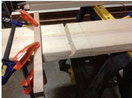
Traçage du second tenon de chaque pied. Les pieds sont 2 2"x6" (4cm x 14cm)
